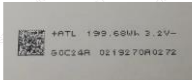
电芯标签 Cell label
